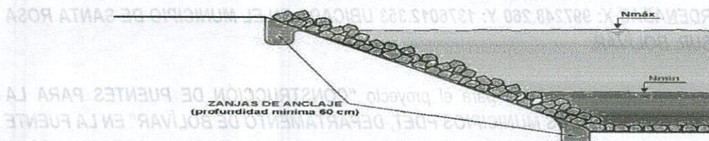
Figura: Protección tipo escollera
