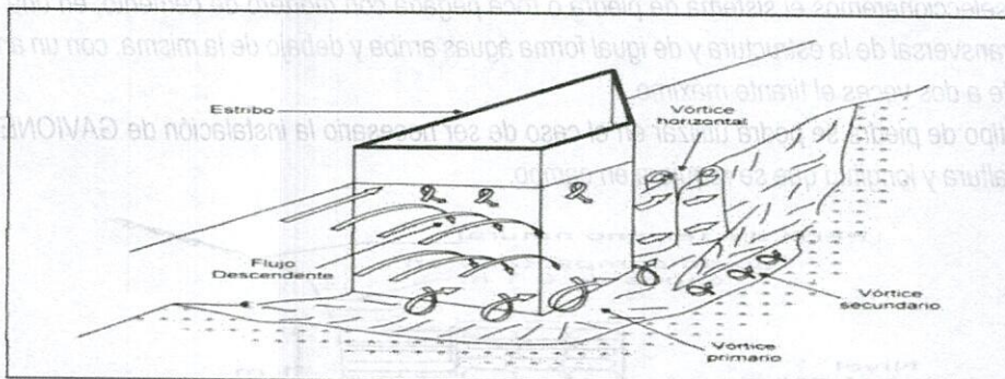
Figura: Socavación local de un estribo
