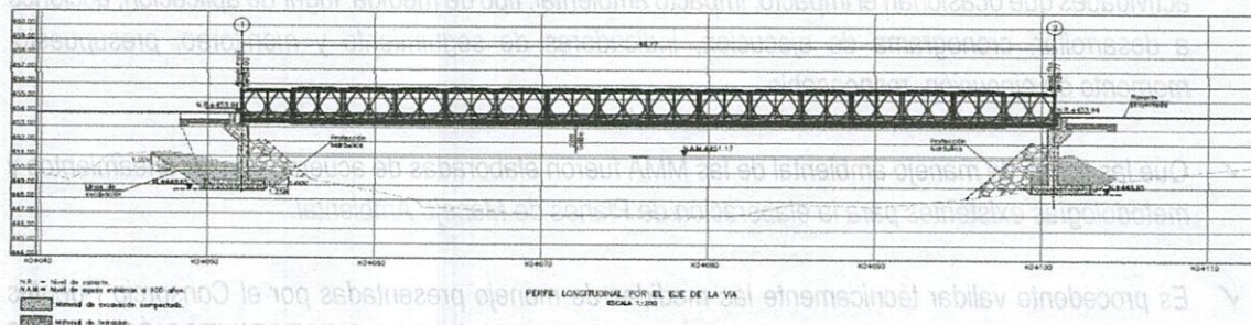
Figura: Perfil de la obra a ejecutar.
