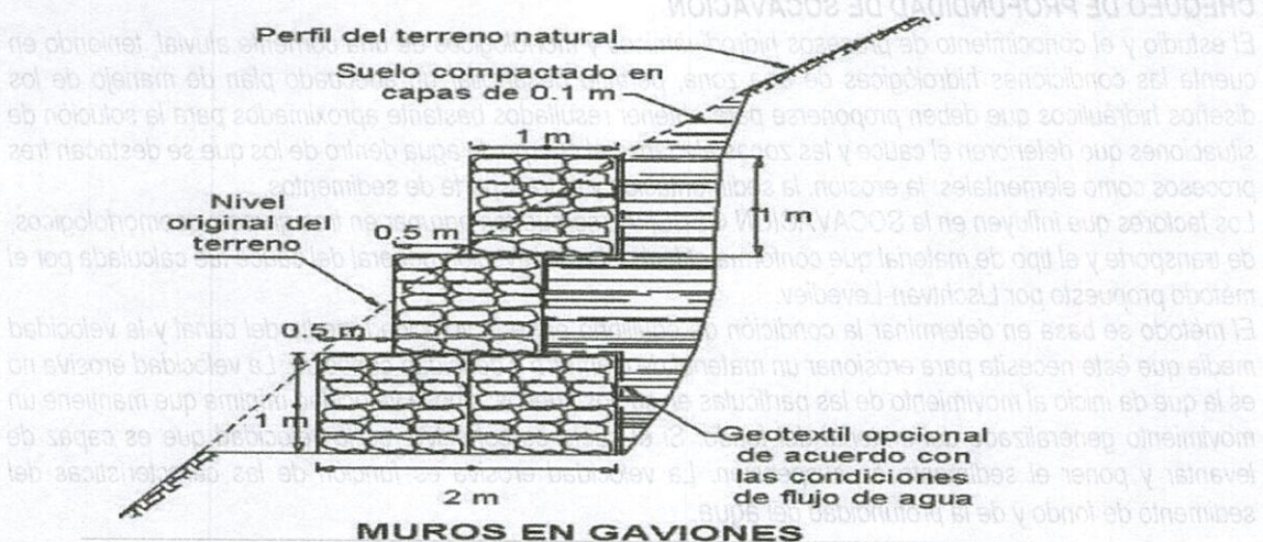
Figura: Esquema típico de muros de gaviones protección cauce.
