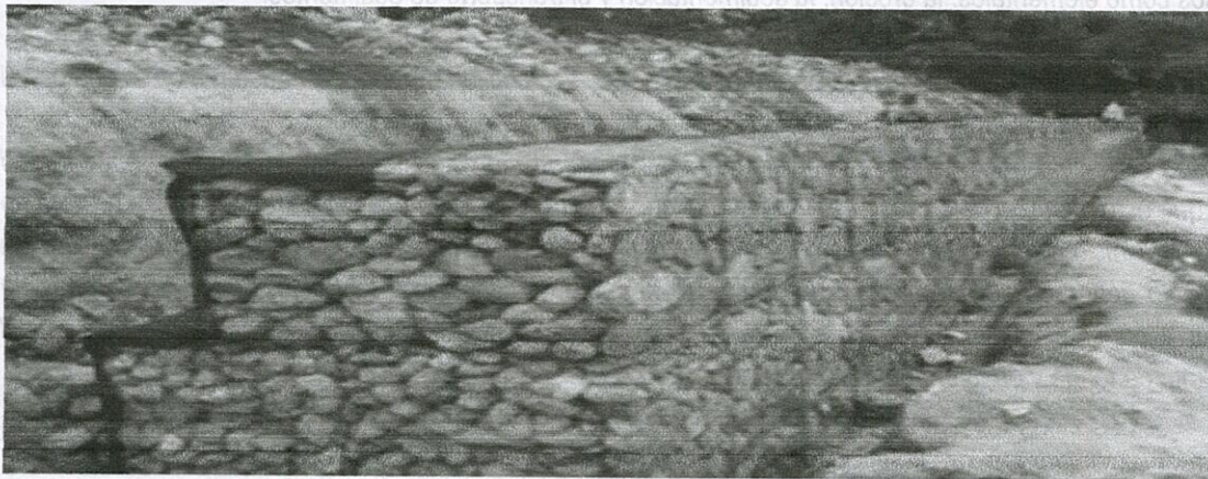
Figura: Gaviones típicos
