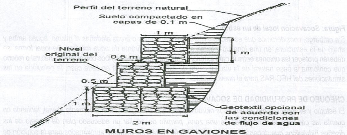
Figura: Esquema típico de muros de gaviones protección cauce.
