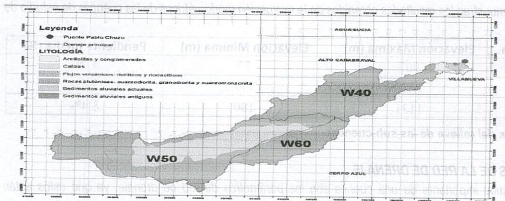
Figura. Formaciones geológicas de la zona de estudio
