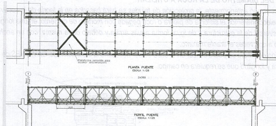
Figura: Perfil de la obra a ejecutar.
