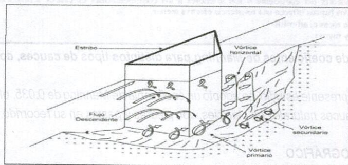
Figura: Socavación local de un estribo
