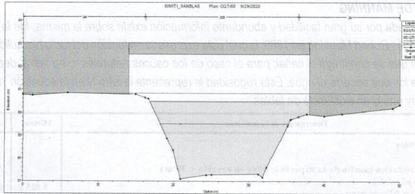
Figura: Sección del cauce en la estación del puente propuesto: 24 m
