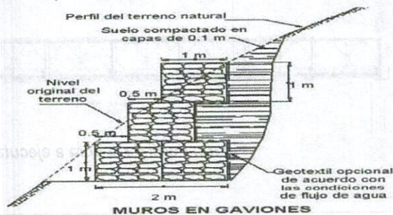
Figura: Esquema típico de muros de gaviones protección cauce
